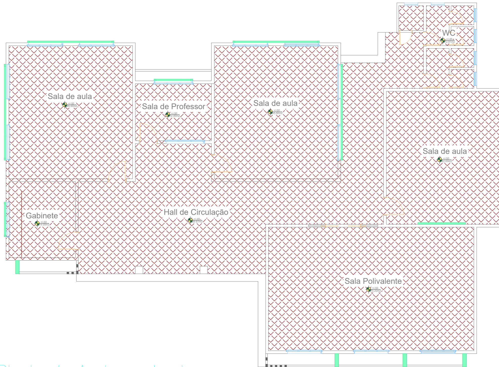
Planta de Acabamento do Pavimento
